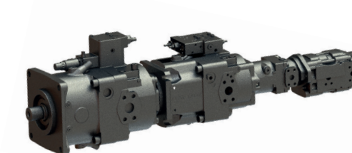
HYDRAULISCHE POMPEN VOOR AANDRIJVING VAN DE POMPGROEP
