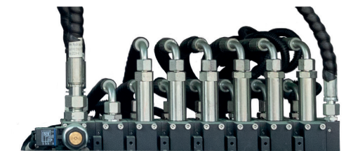
PROPORTIONEEL HYDRAULISCH VERDEELBLOK VAN DE GIEK
