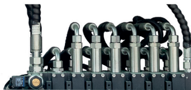
HYDRAULISCH GIEK VERDEELBLOK
